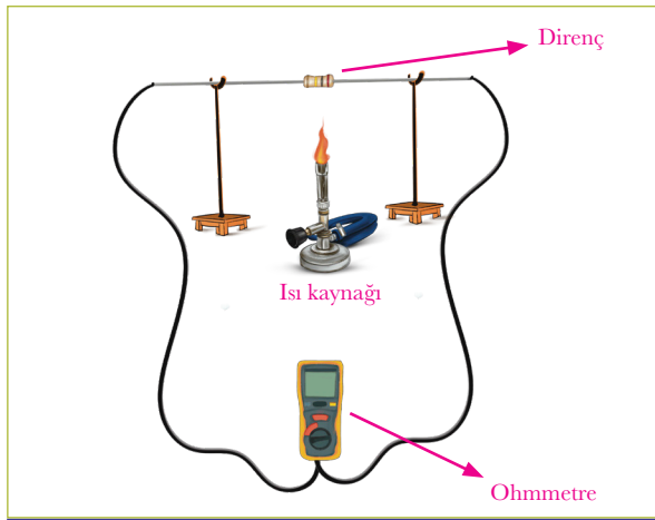
Görsel 3.1: Deney düzeneği
