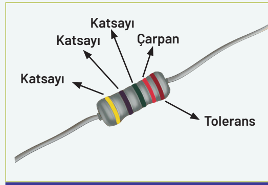
Görsel 3.3: 5 Renkli Direnç
