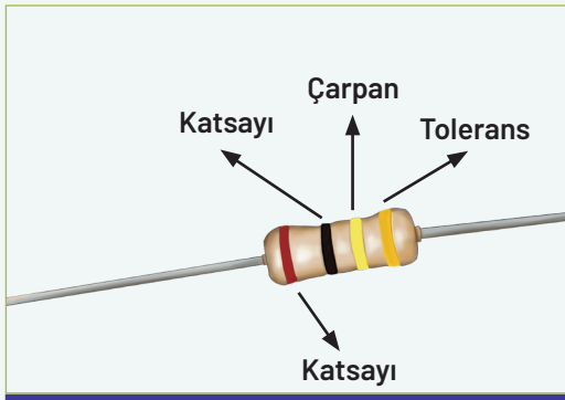
Görsel 3.2: 4 Renkli Direnç
