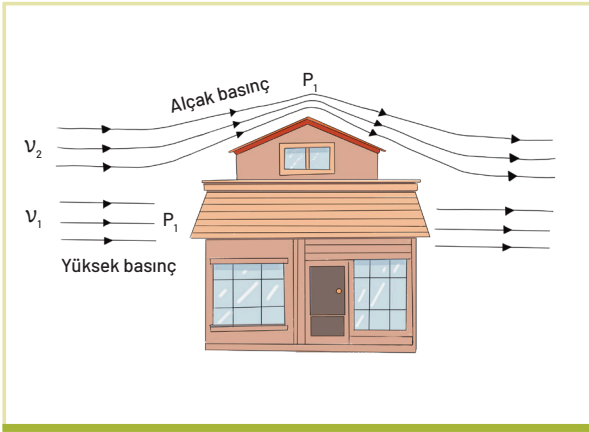
Görsel 3.3: Fırtınalı havalarda evlerin çatısının uçması
