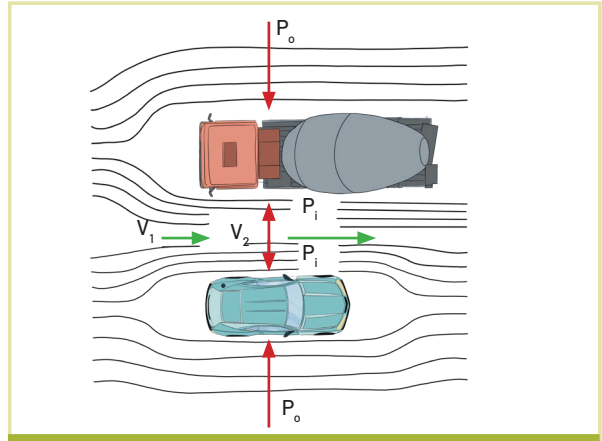
Görsel 3.6: Seyir hâlindeki iki aracın yan yana geçtikleri sırada birbirlerine doğru çekilmesi
