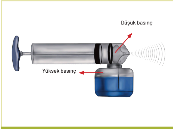
Görsel 3.7: İlaçlama pompasının çalışma ilkesi
