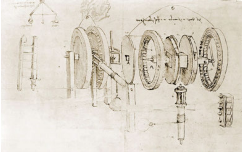
Görsel 3.2: Leonardo da Vinci’nin notlarından alınan bir makine tasarımı
