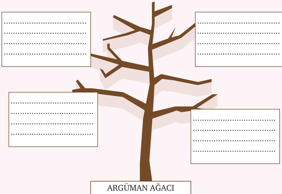
Şekil 2.5: Argüman ağacı
