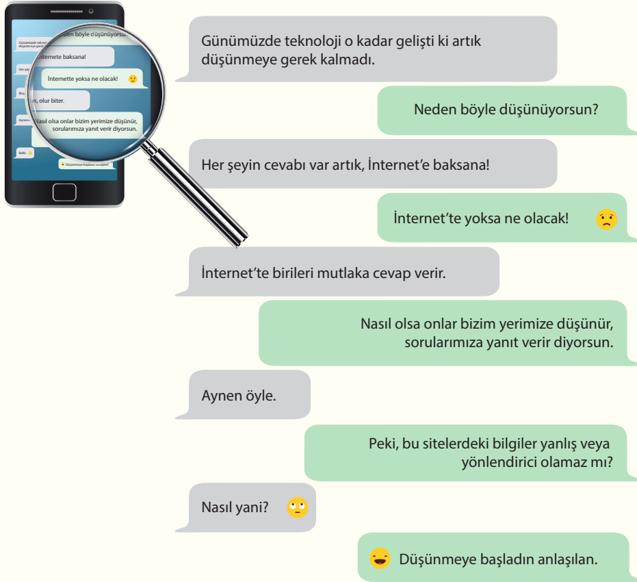
Şekil 1.1: Mesajlaşma
