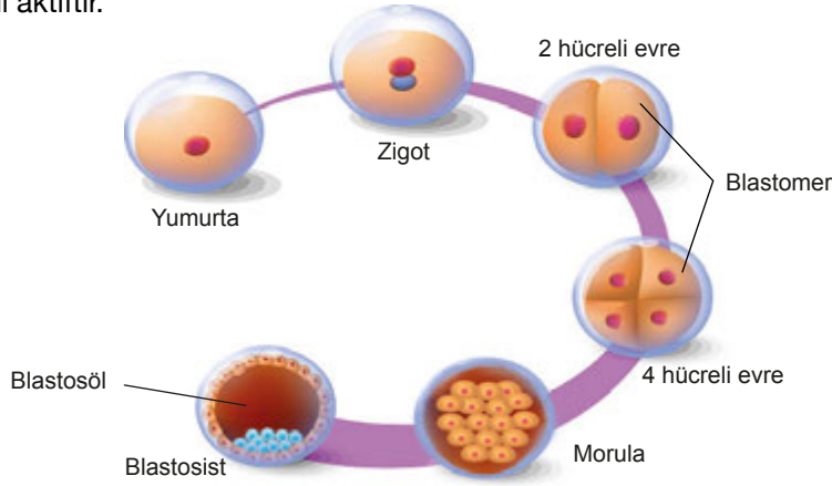
Görsel 1.125: Segmentasyon
