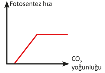
Grafik 2.4: \text{CO}_2 yoğunluğunun fotosentez hızına etkisi
