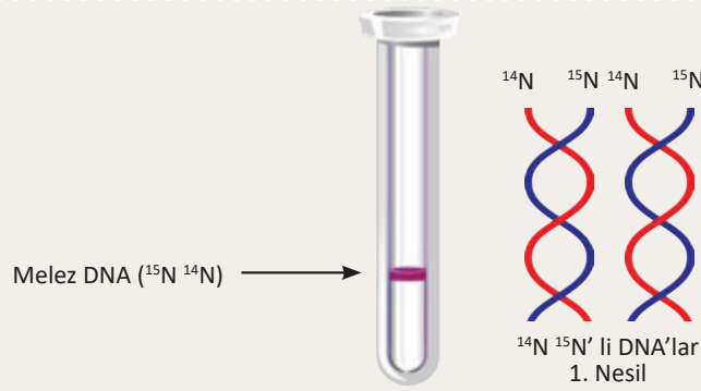
Görsel 1.36: ^{14}\text{N}^{15}\text{N} içeren melez DNA
